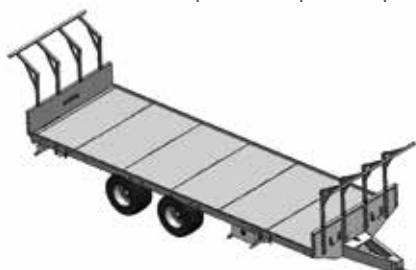
Disegno rimorchio senza rampe con imperiali tipo A
